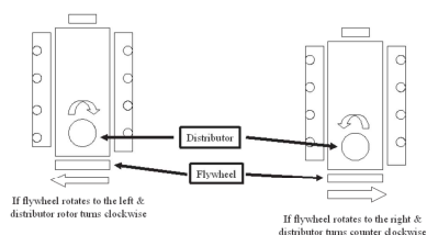
CCW Rotation
