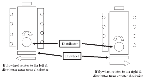
CCW Rotation
